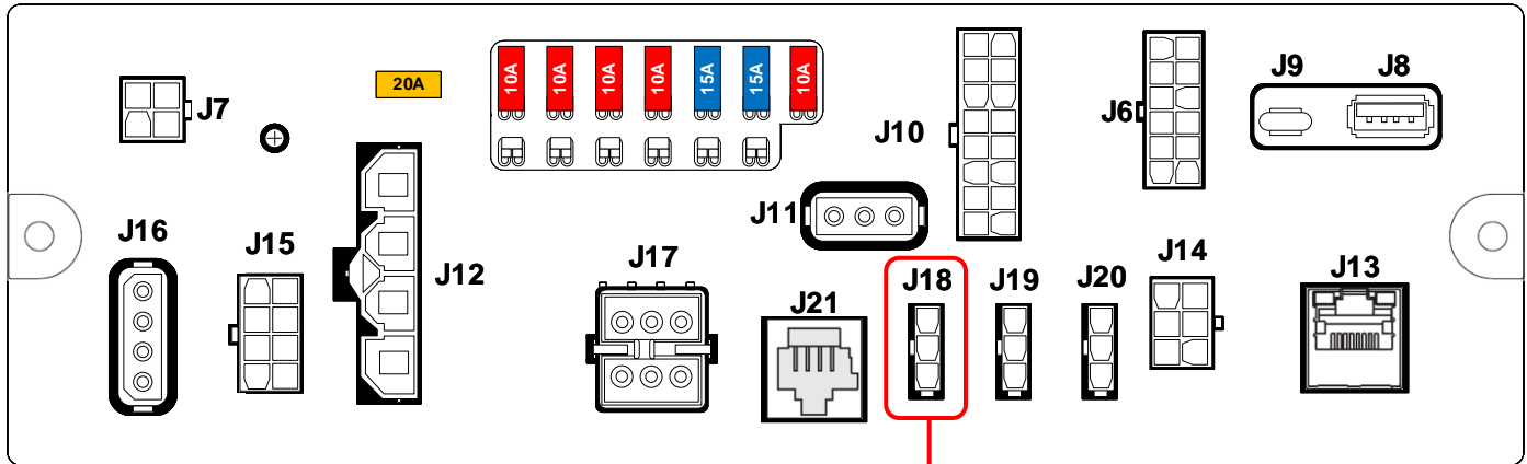
J18 – DATA
